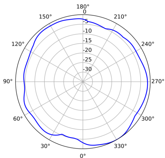
5GHz (Horizontal)
