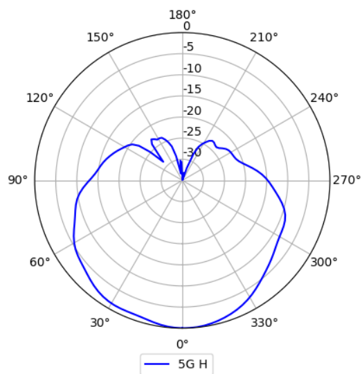
5GHz (Horizontal)
