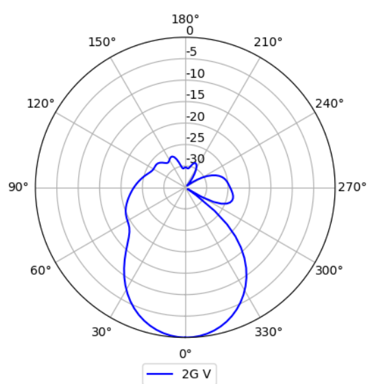
2.4GHz (Vertical)
