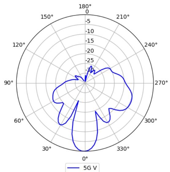
5GHz (Vertical)
