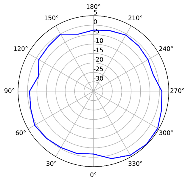
2.4GHz (Vertical)
