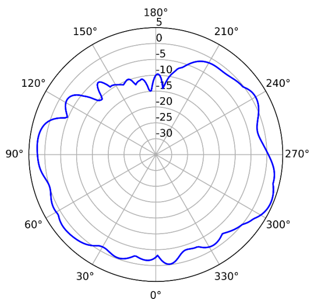
6GHz (Vertical)
