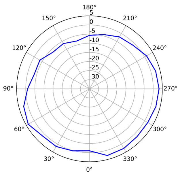
5GHz (Vertical)
